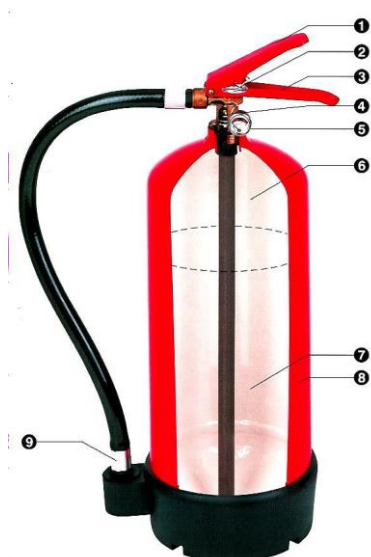
Budowa gaśnicy typu x
